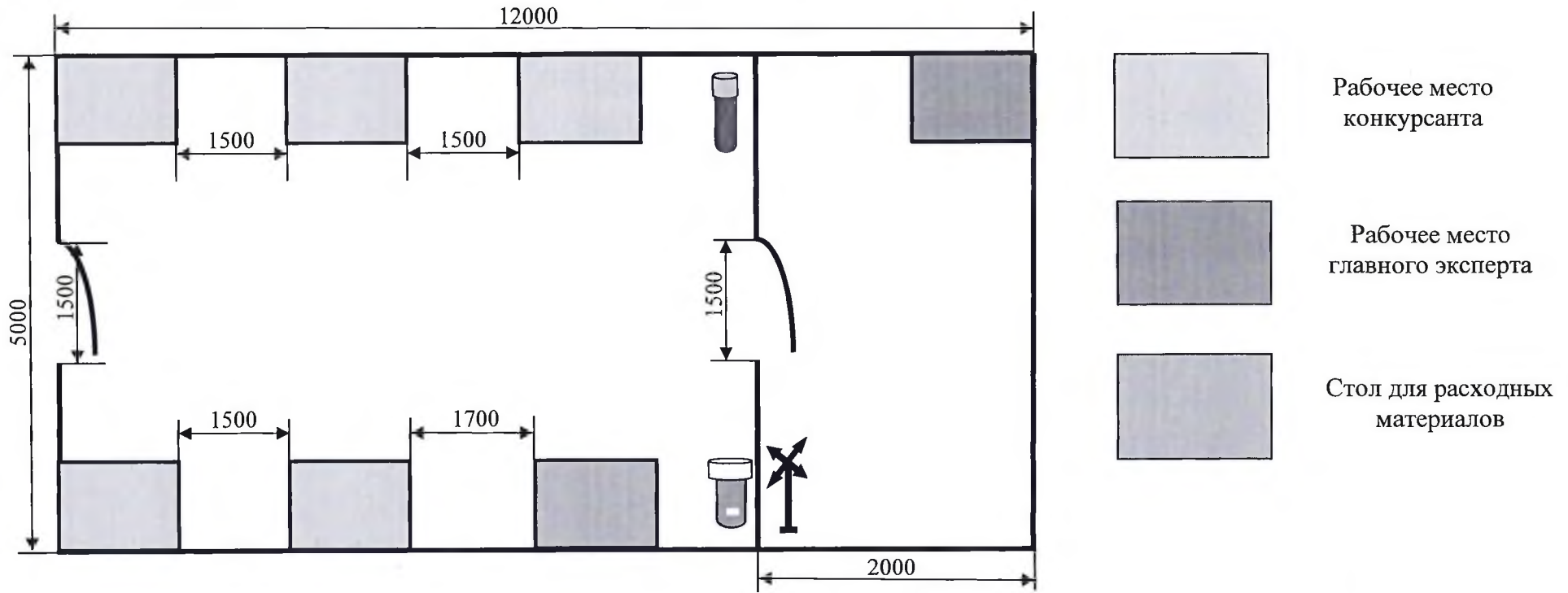
План застройки рабочего места конкурсанта
