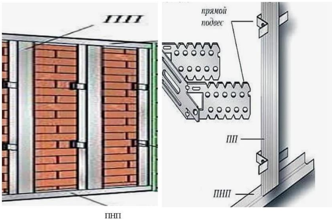
Сборка каркаса
